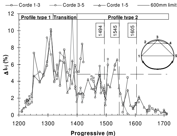
Figure 9 - Déformations mesurées au niveau des capteurs 1-3, 3-5 et 1-5, à 15 m du front dans la phase 1
