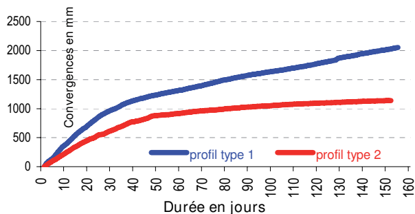
Figure 4 - Cours d'évolution de convergences
