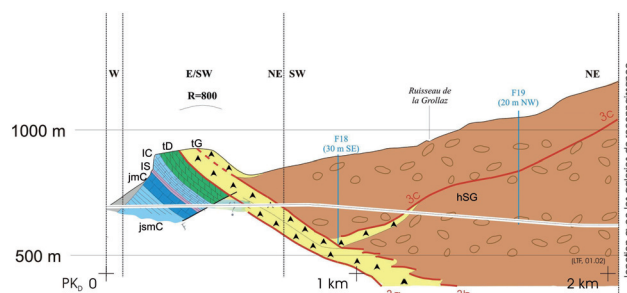
Figure 1 - Coupe géologique
