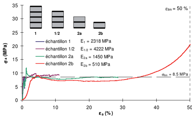
Figure 11 - Courbe caractéristique obtenue en laboratoire lors de la mise en charge mono-axiale de l'élément déformable
