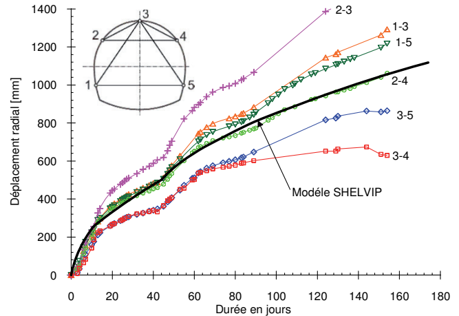
Figure 13 - Comparaison du comportement prévu et observé au cours de l'excavation. Auscultation de la section au PM 1311 avec soutènement souple de type 1 (Barla et al., 2008)
