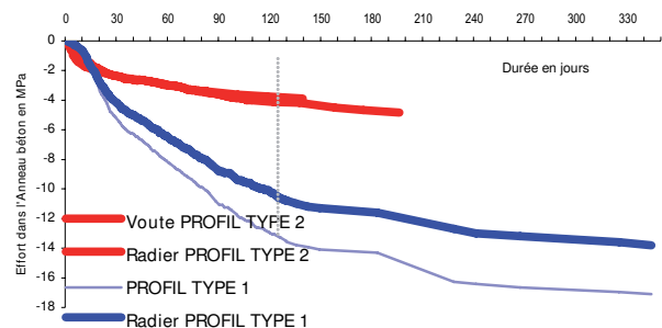
Figure 8 - Courbes d'évolution de la mise en charge de l'anneau béton
