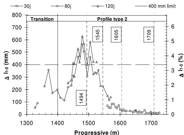
Figure 10 - Convergences observées à 30, 80 et 120 jours suivant l'excavation après mise en œuvre de la phase 2
