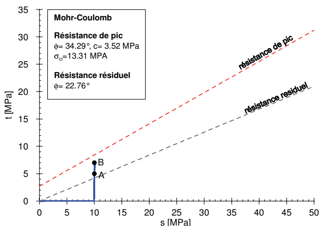
Figure 12 - Comparaison du comportement prévu (modèles SHELVIP) et mesuré en laboratoire (Barla et al., 2008)
